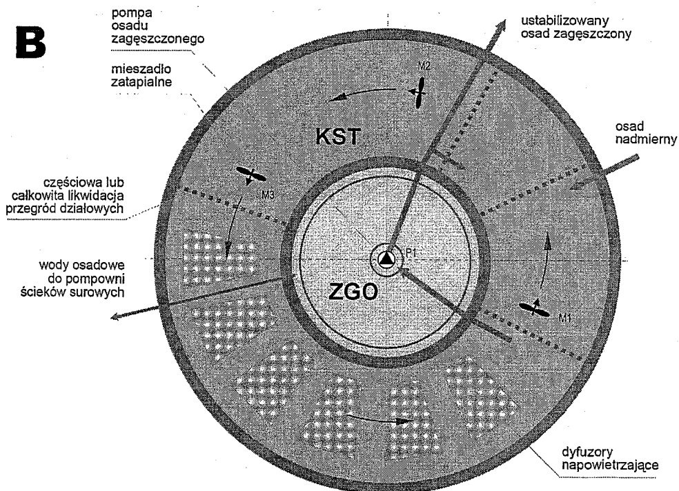
A - Blok reaktora przed modernizacją B - Blok reaktora po modernizacji
